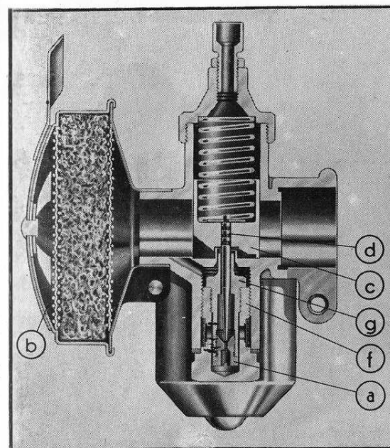
Obr. 15 Řez splynovače.
