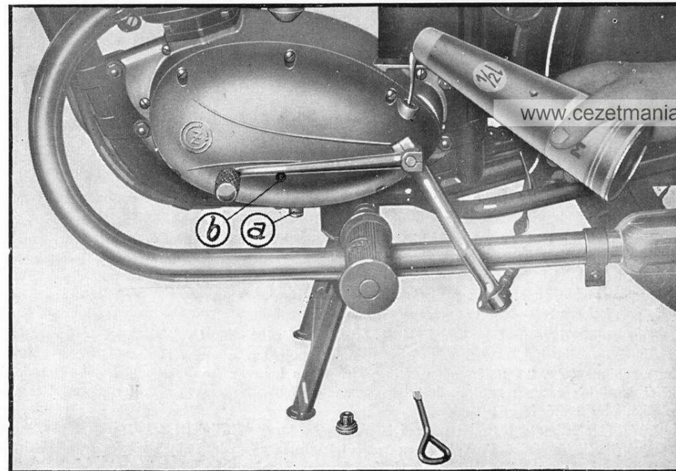
Obr. 7 Mazání motocyklu
