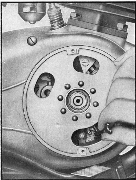
Obr. 20 Seřízení předstihu
