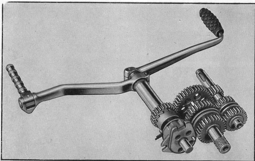
Obr. 18 Převodové ústrojí
