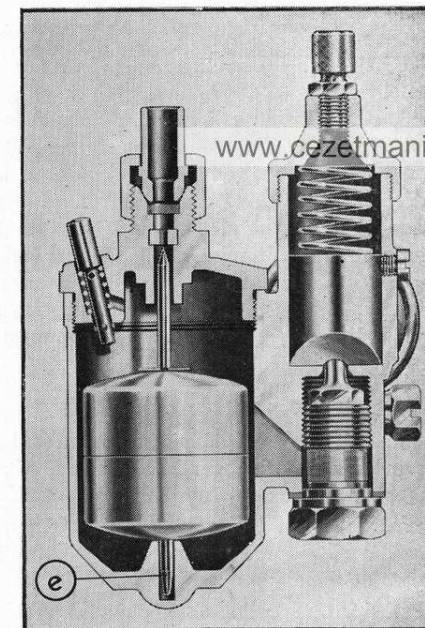
Obr. 15a Řez splynovače.
