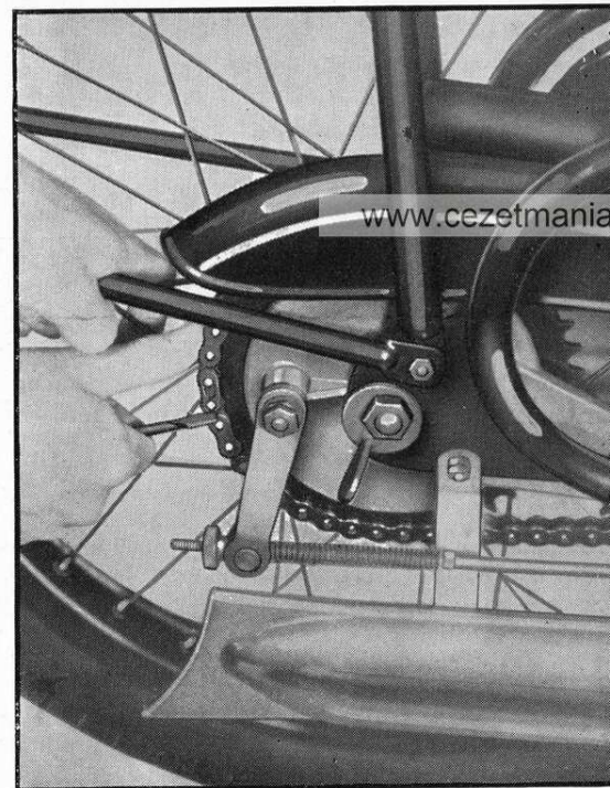
Obr. 8 Rozepínání řetězu
