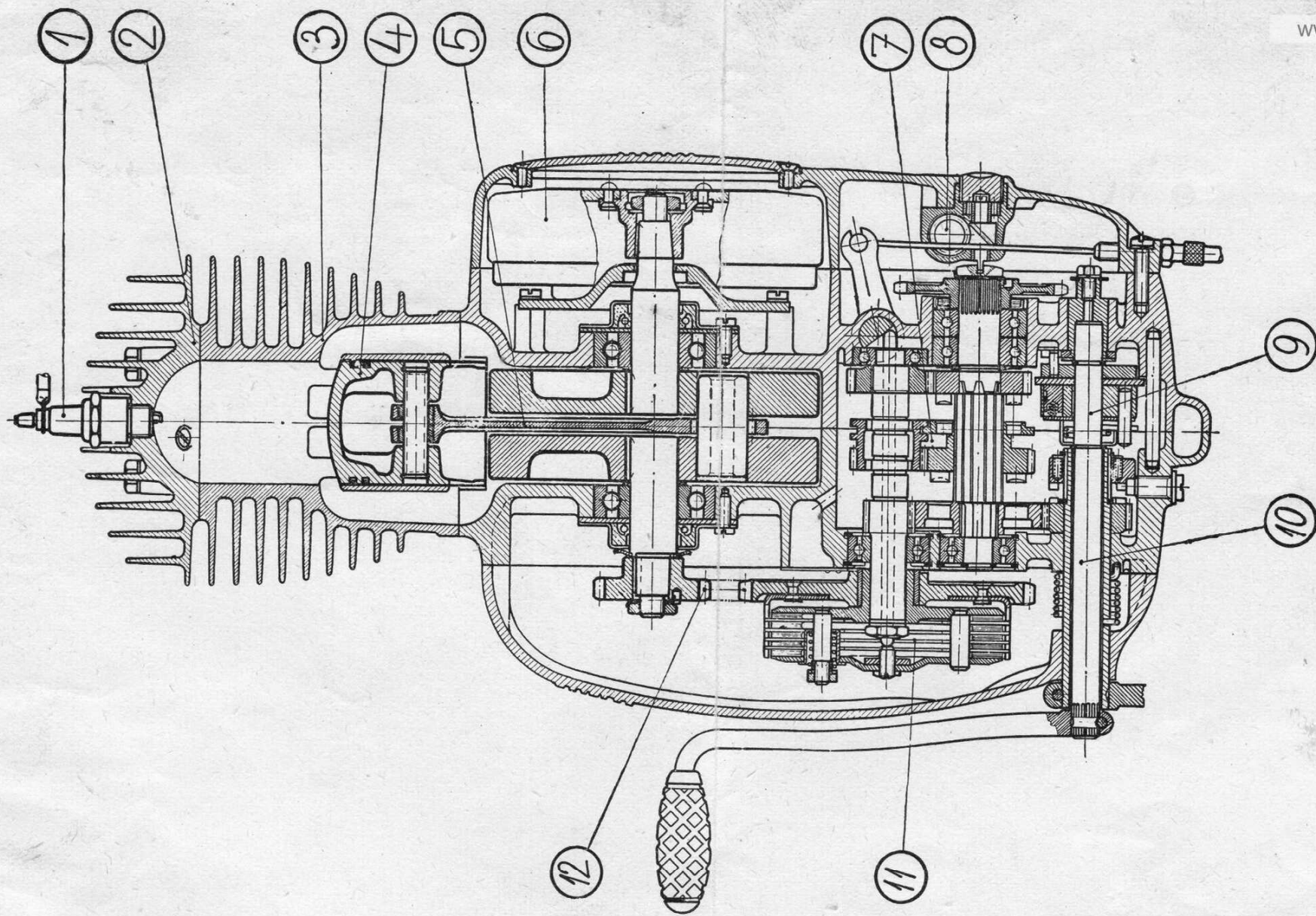
Obr. 21 Řez motoru
