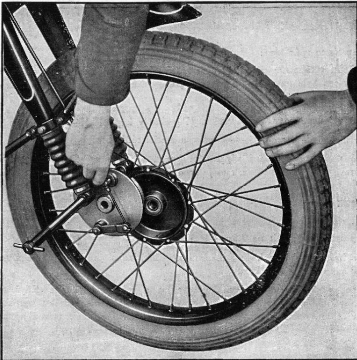
Obr. 10 Vyjímání předního kola
