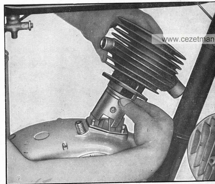
Obr. 14 Nasazování válce
