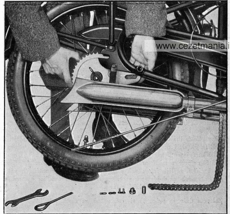
Obr. 11 Vyjímání zadního kola
